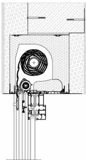
Rolluik – SKB
