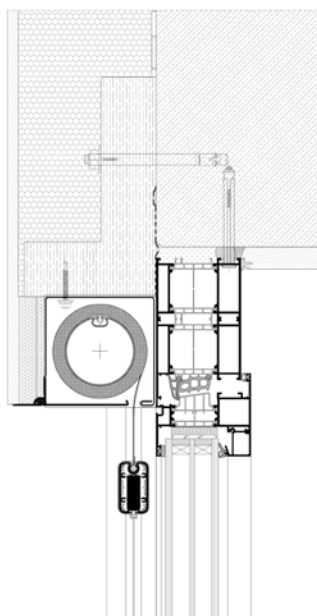
inbouwversie
