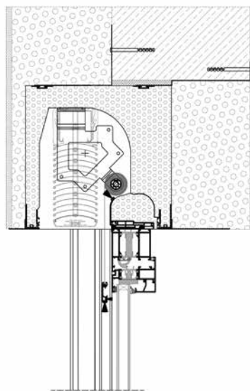
buitenjaloezieënzijn - SKB
