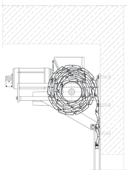
Roldeur – BPR/KNJ
