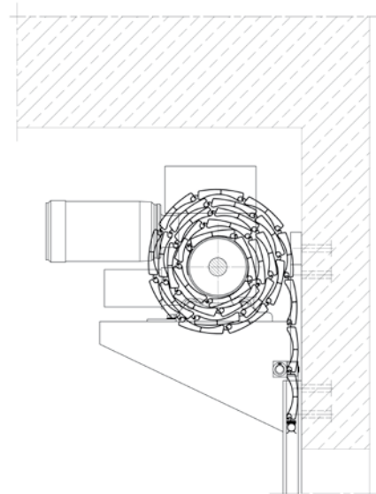
Roldeur – BPR/KNS
