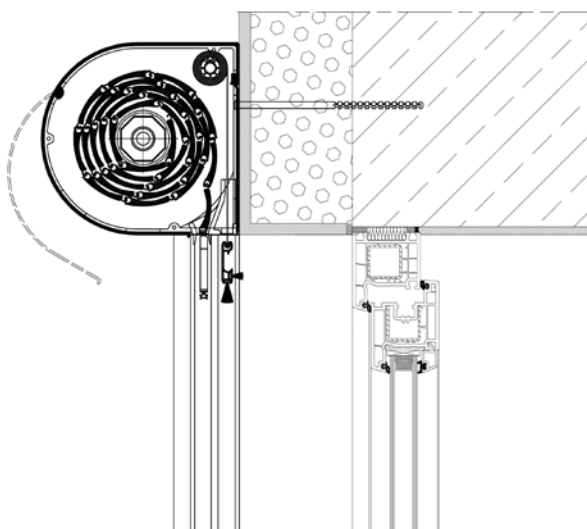
Rolluik – SKO
