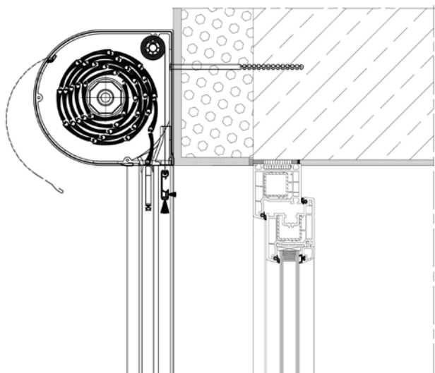
Rolluik – SKO-P
