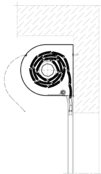
Roldeur – BGR/SKO-P
